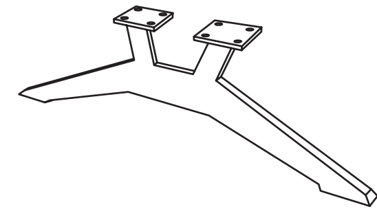
Schwertkufe 750x230 mm Sword skid 750x230 mm
