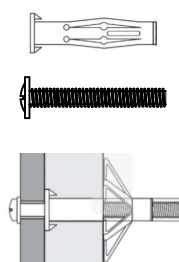
Hohlraum Metalldübel
