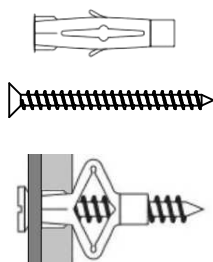
Hohlraum Kunststoffdübel
