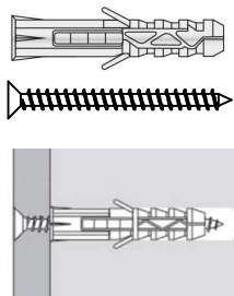
Cheville nylon "Fischer"
