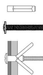
Hohlraumdübel "Molly"
